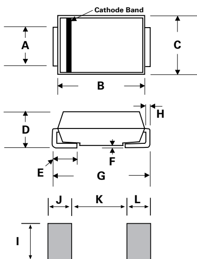
DO-214AC (SMA)
