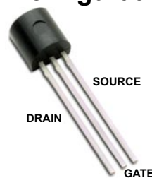
TO-92 (N3)
